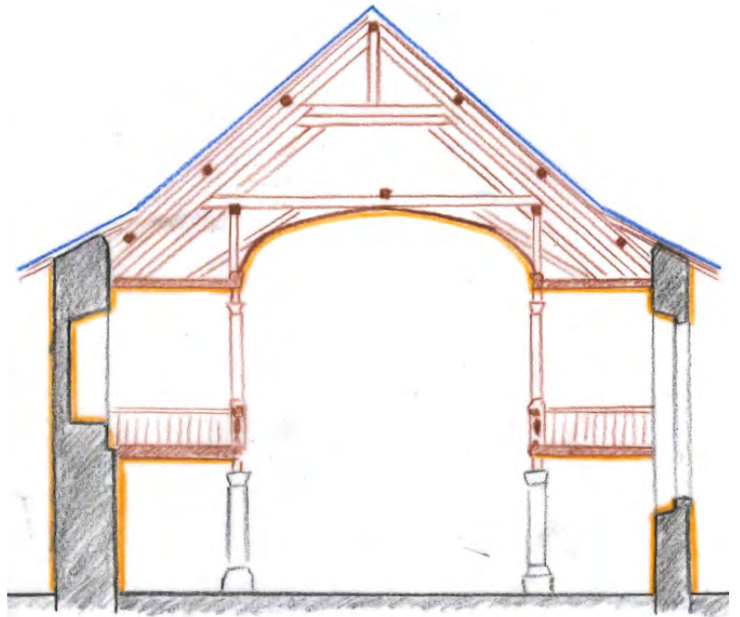
Coupe sur la nef
