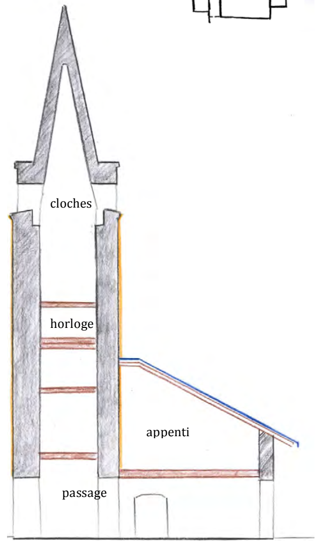
Coupe sur le clocher
